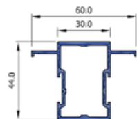
Glazing Bar SF44029
