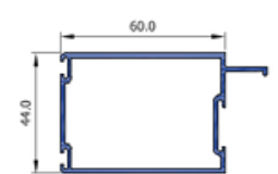
R11 (W) Door Stile 60 (R3 60) SF44021
