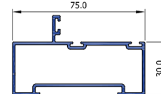
Folding Door Jamb FD03
