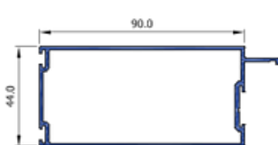
R9 (W) Door Stile 90 (R3 90) SF44041
