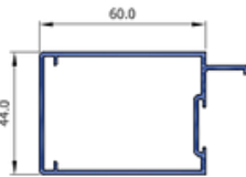
R11 Door Stile 60 (R1 60) SF44020
