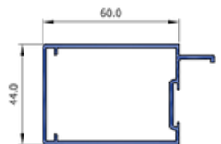
R11 Door Stile 60 (R1 60) SF44020
