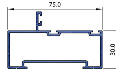
Folding Door Jamb FD03
