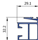
Patio Slider Interlocker
